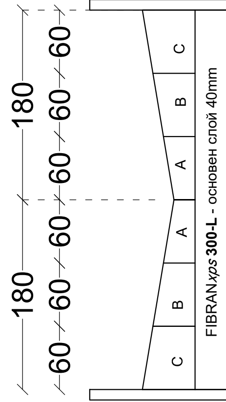
Разрез A-A
